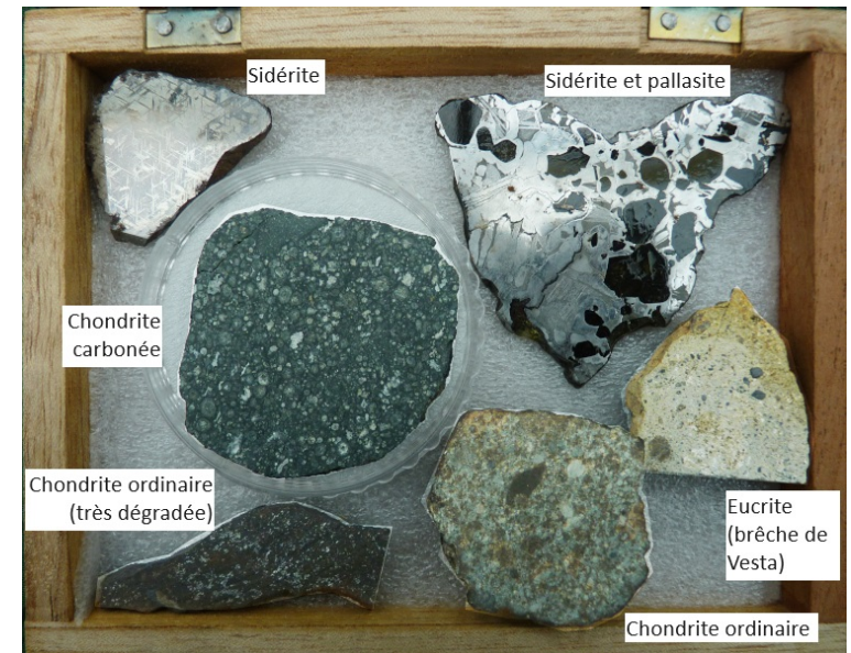
Quelques échantillons de météorites
